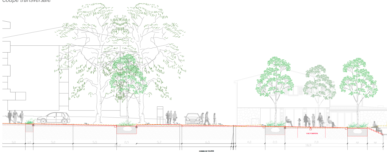
Coupe transversale
